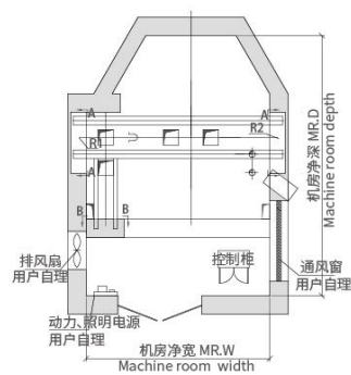
机房平面布置图 Machine room plan
