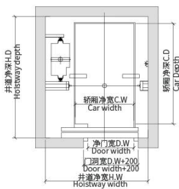
井道平面布置图 hoistway plan
