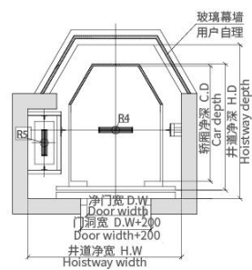
井道平面布置图 Hoistway plan
