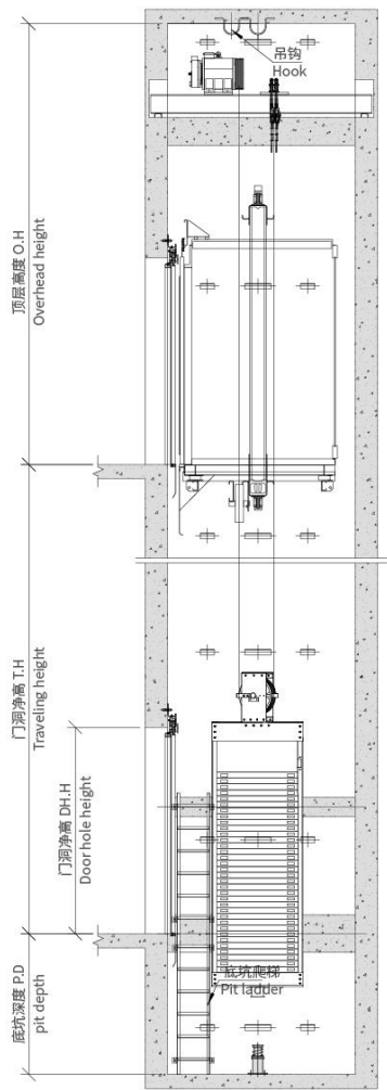
井道立面布置图 Hoistway section
