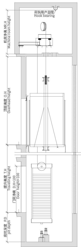
井道立面图 Hoistway section
