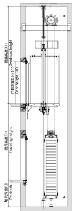
井道立面图 Hoistway section
