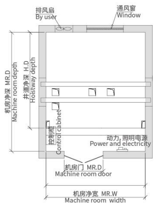
机房平面布置图 Machine room plan
