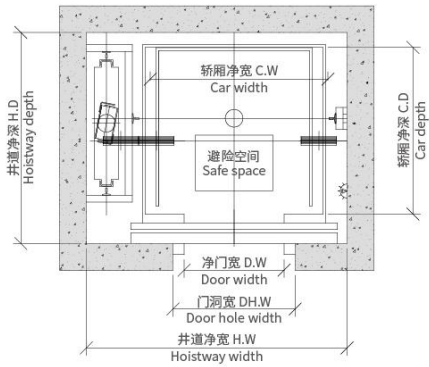
630-1150KG 井道平面布置图 Hoistway plan
