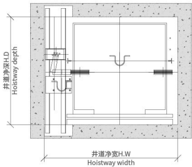
轿底轮结构 顶层平面布置图 Overhead floor plan
