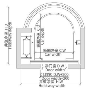
井道平面布置图 Hoistway plan
