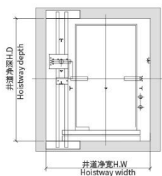
顶层平面图 Overhead floor plan
